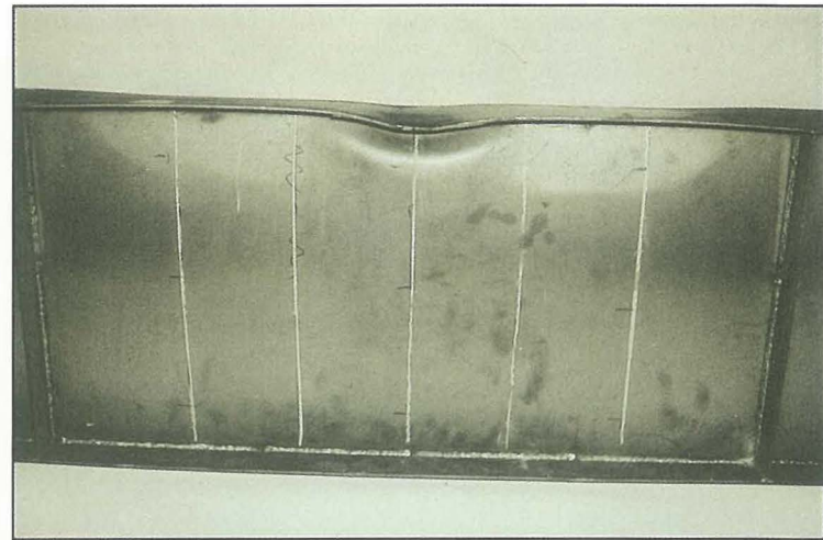
Слика 1 – Експериментално испитивање стабилности челичних лимених носача
