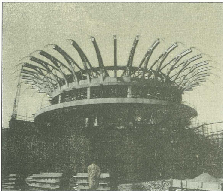
Слика 4 – Музеј ваздухопловства на Аеродрому Београд
